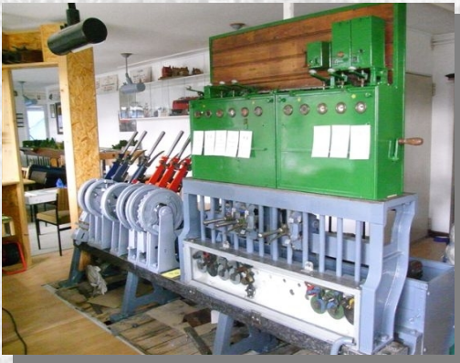
Historisches Hebel- und Blockwerk
